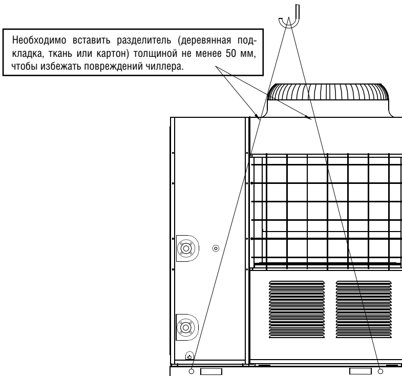
Рис. 2-1. Подъем модуля
